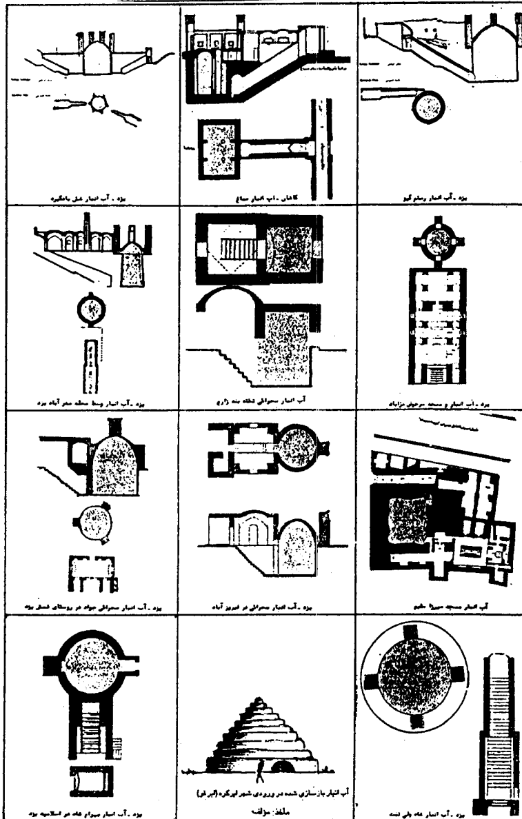
ورودی □ خزینة ■ بادگیر ■ شکل ۱: جزئیات آب انبارها
